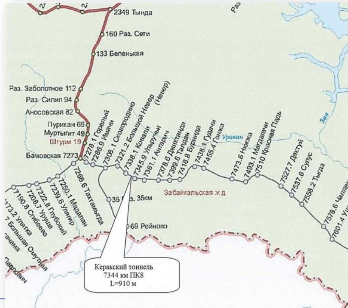
Расположение существующего Керакского тоннеля
